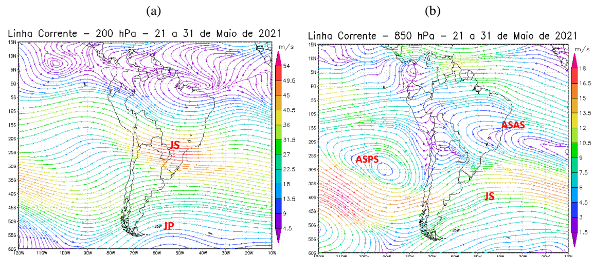
Figura 8 - Campos de Linha de Corrente 200 hPa. - (a) e 850 hPa. - (b), do 3º Decêndio de maio de 2021; demonstrando interação entre os sistemas atmosféricos: Jato Subtropical (JS), Anticiclone Subtropical do Atlântico Sul (ASAS) e Anticiclone Subtropical do Pacífico Sul (ASPS).
