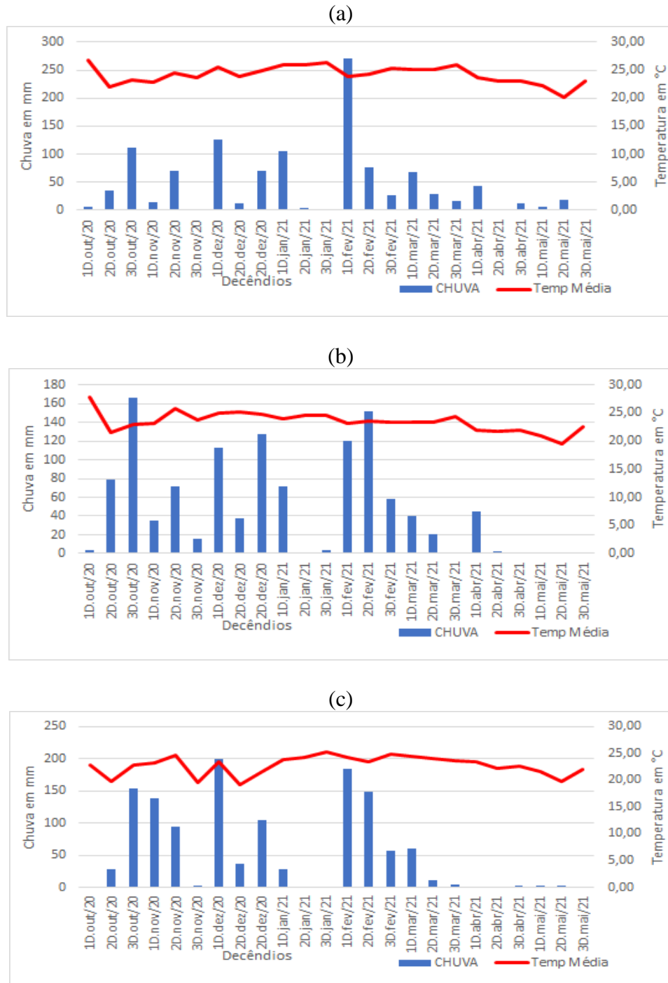
Figura 3: Histograma de Chuva e Temperatura: Caratinga (a); Timóteo (b) e PERD (c) – (outubro/2020 a maio/2021).
