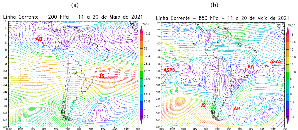
Figura 7 - Campos de Linha de Corrente 200 hPa. - (a) e 850 hPa. - (b), do 2º Decêndio de maio de 2021; demonstrando interação entre os sistemas atmosféricos: Alta da Bolívia (AB), Bloqueio Atmosférico (BA), Jato Subtropical (JS), Anticiclone Subtropical do Atlântico Sul (ASAS), Anticiclone Subtropical do Pacífico Sul (ASPS) e o Anticiclone Polar (AP).
