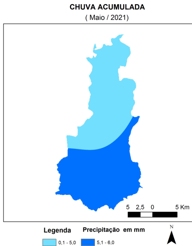
Figura 5 - Espacialização da Chuva da Acumulada em maio de 2021. FONTE dos Dados: INMET e INPE
