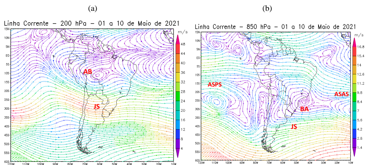
Figura 6 - Campos de Linha de Corrente 200 hPa. - (a) e 850 hPa. - (b), do 1º Decêndio de maio de 2021; demonstrando interação entre os sistemas atmosféricos: Alta da Bolívia (AB), Bloqueio Atmosférico (BA), Jato Subtropical (JS), Anticiclone Subtropical do Atlântico Sul (ASAS) e Anticiclone Subtropical do Pacífico Sul (ASPS).
