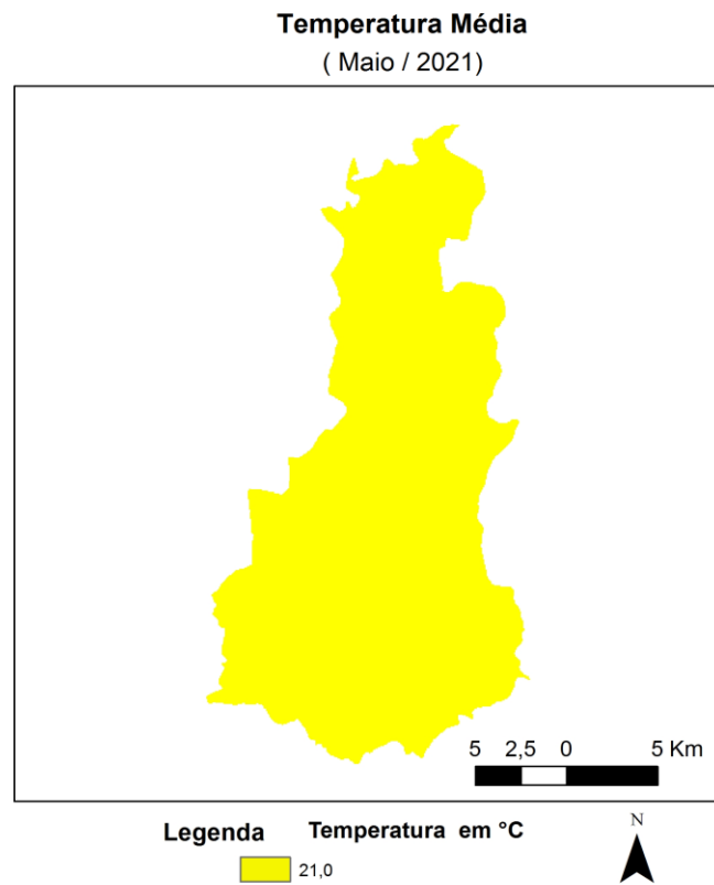
Figura 4 - Espacialização da Temperatura Média em maio de 2021. FONTE dos Dados: INMET e INPE
