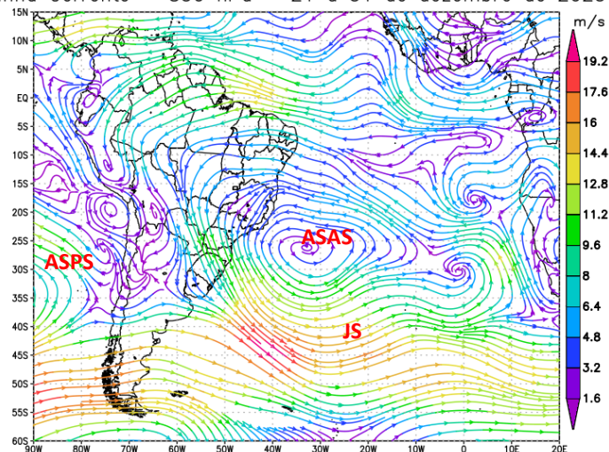
Figura 8 - Campos de Linha de Corrente 200 hPa (a), 500 hPa (b) e 850 hPa (c), do 3º Decêndio de dezembro de 2025; demonstrando interação entre os sistemas atmosféricos: Jato Subtropical (JS), Alta da Bolívia, Vórtice Ciclônico de Altos Níveis (VCAN), Anticiclone Subtropical do Atlântico Sul (ASAS) e Anticiclone Subtropical do Pacífico Sul (ASPS). FONTE - Dados: NOAA 2025.
