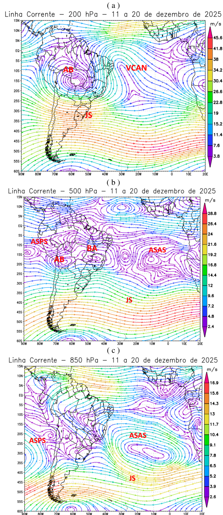
Figura 7 - Campos de Linha de Corrente 200 hPa (a), 500 hPa (b) e 850 hPa (c), do 2º Decêndio de dezembro de 2025; demonstrando interação entre os sistemas atmosféricos: Jato Subtropical (JS), Alta da Bolívia (AB), Vórtice Ciclônico de Altos Níveis (VCAN), Bloqueio Atmosférico (BA), Anticiclone Subtropical do Atlântico Sul (ASAS) e o Anticiclone Subtropical do Pacífico Sul (ASPS).
