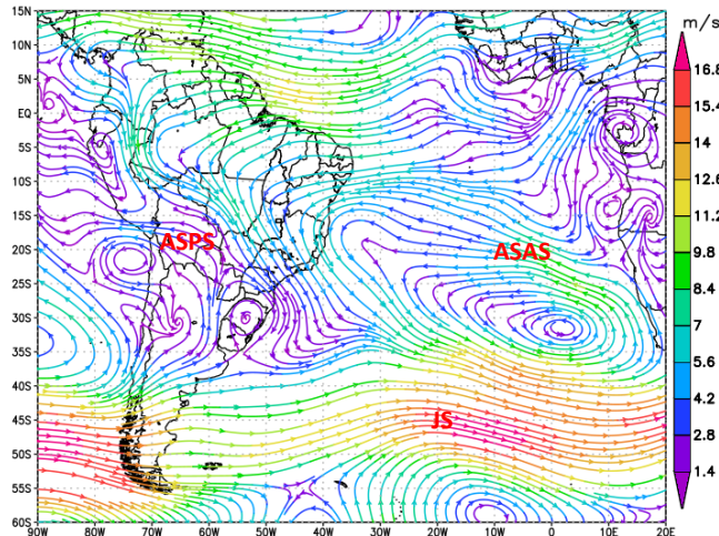
Figura 6 - Campos de Linha de Corrente 200 hPa (a), 500 hPa (b) e 850 hPa (c), do 1º Decêndio de dezembro de 2025; demonstrando interação entre os sistemas atmosféricos: Jato Subtropical (JS), Alta da Bolívia (AB), Vórtice Ciclônico de Altos Níveis (VCAN), Anticiclone Subtropical do Atlântico Sul (ASAS) e o Anticiclone Subtropical do Pacífico Sul (ASPS).
