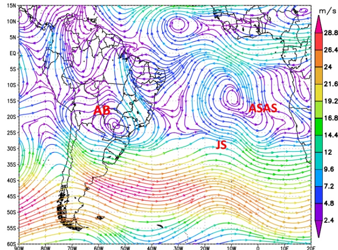
(c) Linha Corrente – 850 hPa – 21 a 31 de dezembro de 2025
