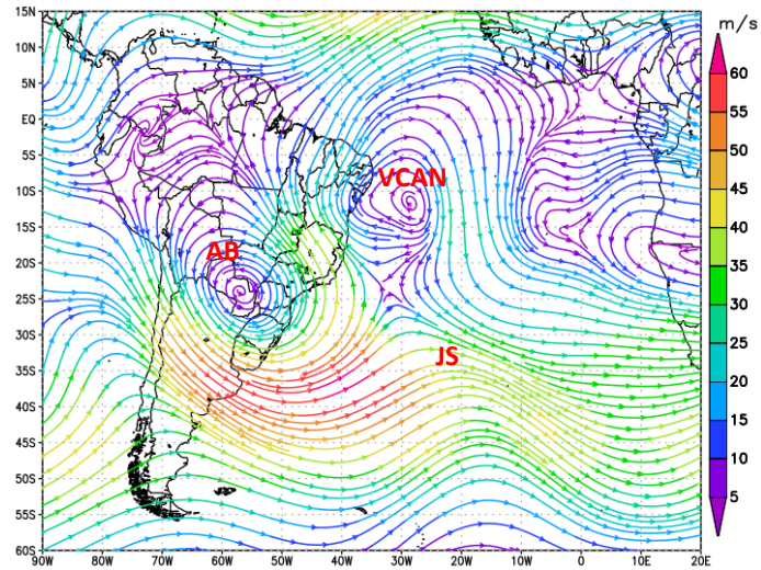
(b) Linha Corrente – 500 hPa – 21 a 31 de dezembro de 2025
