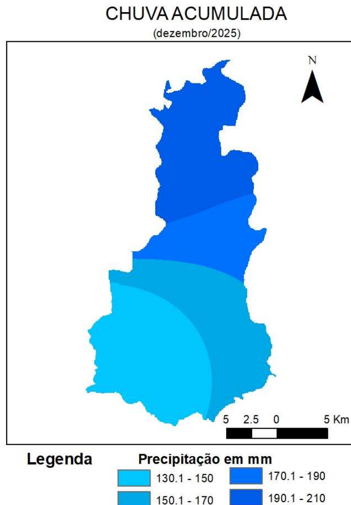
Figura 5 - Espacialização da Chuva da Acumulada em dezembro de 2025. FONTE dos Dados: INMET e INPE
