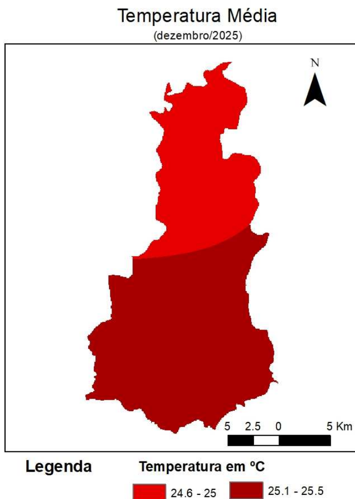
Figura 4 - Espacialização da Temperatura Média em dezembro de 2025. FONTE dos Dados: INMET e INPE
