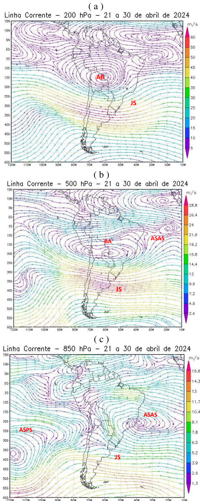
Figura 8 - Campos de Linha de Corrente 200 hPa- (a), 500 hPa - (b) e 850 hPa - (c), do 3º Decêndio de abril de 2024; demonstrando interação entre os sistemas atmosféricos: Jato Subtropical (JS), Alta da Bolívia (AB), Bloqueio Atmosférico (BA), Anticiclone Subtropical do Atlântico Sul (ASAS) e Anticiclone Subtropical do Pacífico Sul (ASPS). FONTE - Dados: NOAA 2024.
