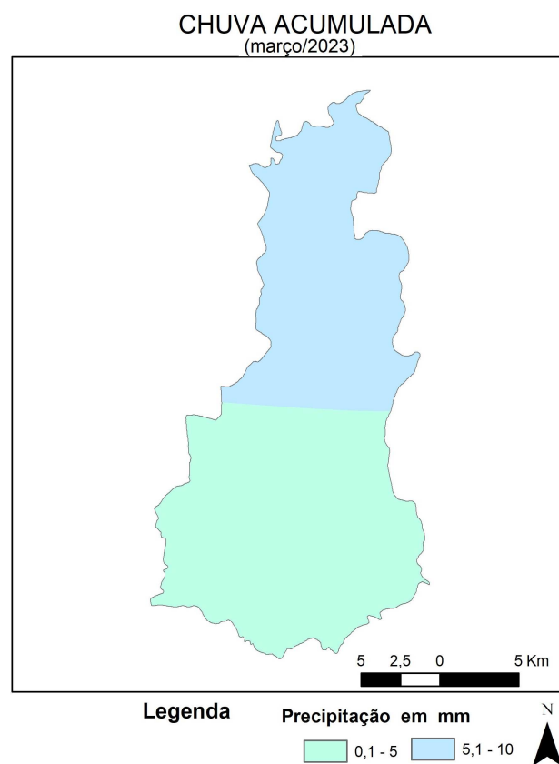
Figura 5 - Espacialização da Chuva da Acumulada em março de 2023. FONTE dos Dados: INMET e INPE
