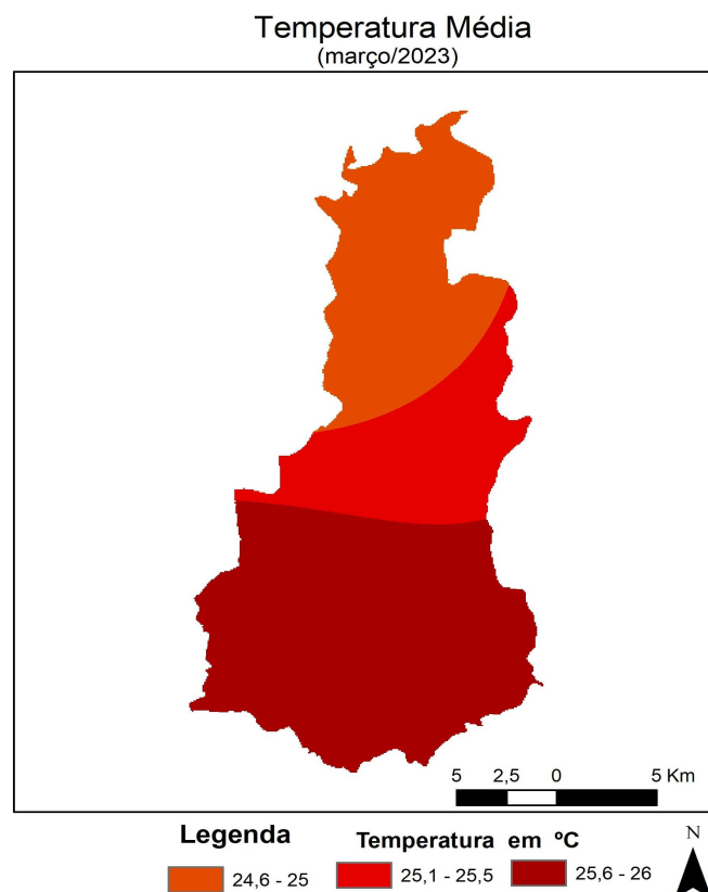
Figura 4 - Espacialização da Temperatura Média em março de 2023. FONTE dos Dados: INMET e INPE
