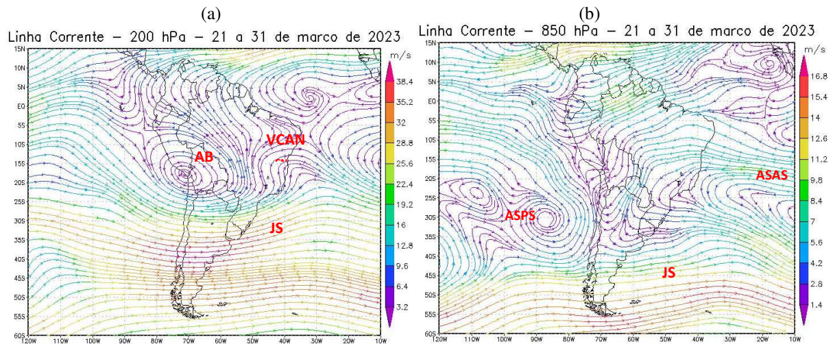
Figura 8 - Campos de Linha de Corrente 200 hPa. - (a) e 850 hPa. - (b), do 3º Decêndio de março de 2023; demonstrando interação entre os sistemas atmosféricos: Jato Subtropical (JS), Alta da Bolívia (AB), Vórtice Ciclônico de Altos Níveis (VCAN), Anticiclone Subtropical do Atlântico Sul (ASAS), Anticiclone Subtropical do Pacífico Sul (ASPS) e Bloqueio Atmosférico (BA).
