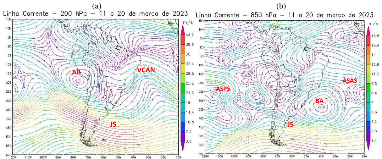
Figura 7 - Campos de Linha de Corrente 200 hPa. - (a) e 850 hPa. - (b), do 2º Decêndio de março de 2023; demonstrando interação entre os sistemas atmosféricos: Jato Subtropical (JS), Alta da Bolívia (AB), Vórtice Ciclônico de Altos Níveis (VCAN), Anticiclone Subtropical do Atlântico Sul (ASAS) e o Anticiclone Subtropical do Pacífico Sul (ASPS) e Bloqueio Atmosférico (BA).
