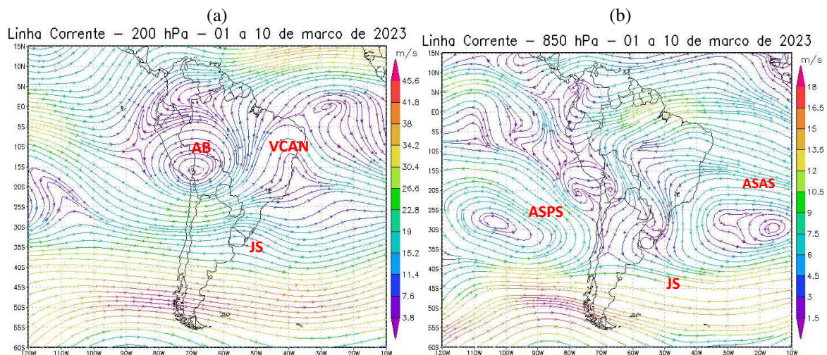
Figura 6 - Campos de Linha de Corrente 200 hPa. - (a) e 850 hPa. - (b), do 1º Decêndio de março de 2023; demonstrando interação entre os sistemas atmosféricos: Jato Subtropical (JS), Alta da Bolívia (AB), Vórtice Ciclônico de Altos Níveis (VCAN), Anticiclone Subtropical do Atlântico Sul (ASAS) e o Anticiclone Subtropical do Pacífico Sul (ASPS).
