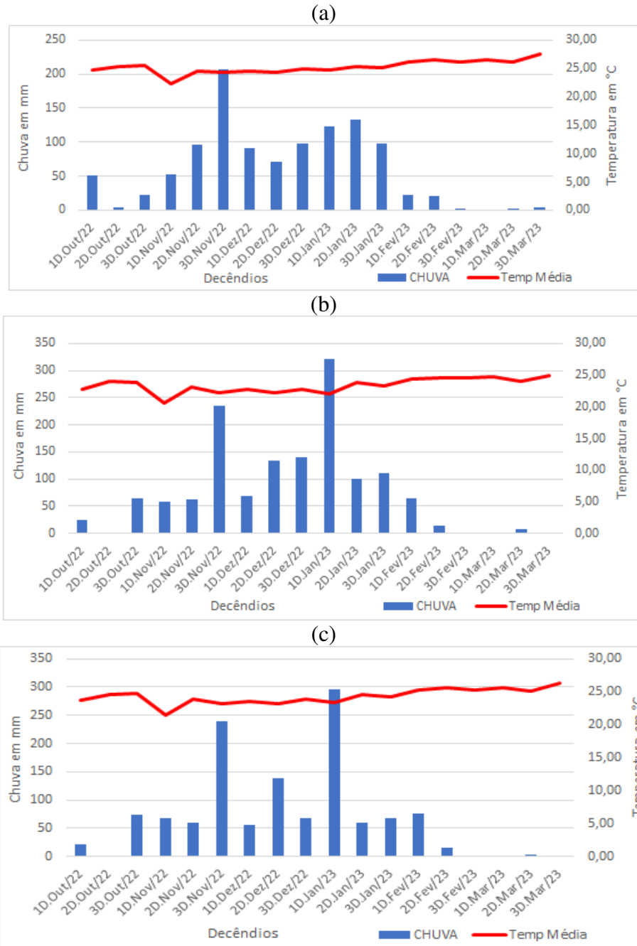
Figura 3: Histograma de Chuva e Temperatura: Caratinga (a); Timóteo (b) e PERD (c) – (outubro de 2022 a março de 2023).
