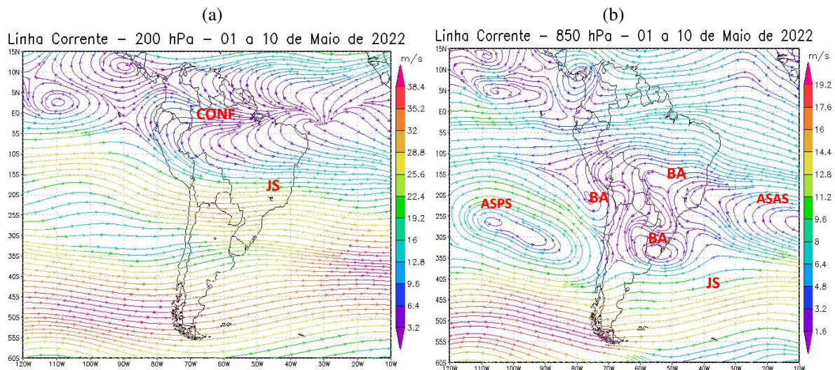
Figura 6 - Campos de Linha de Corrente 200 hPa. - (a) e 850 hPa. - (b), do 1° Decêndio de maio de 2022; demonstrando interação entre os sistemas atmosféricos: Jato Subtropical (JS), Bloqueio Atmosférico (BA), Confluência (CONF) Anticiclone Subtropical do Atlântico Sul (ASAS) e o Anticiclone Subtropical do Pacífico Sul (ASPS).
