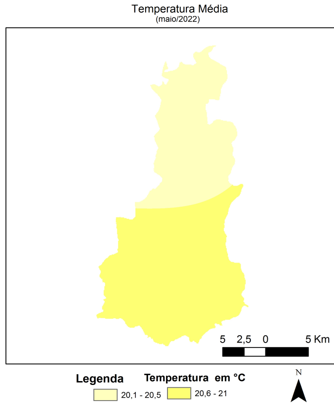
Figura 4 - Espacialização da Temperatura Média em maio de 2022. FONTE dos Dados: INMET e INPE
