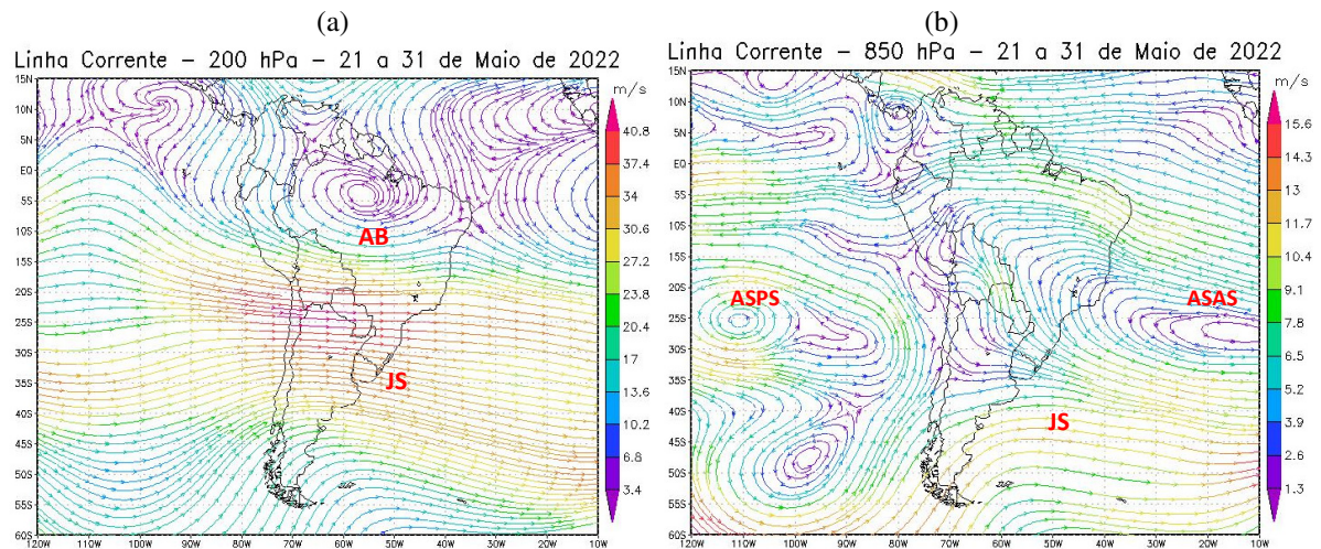
Figura 8 - Campos de Linha de Corrente 200 hPa - (a) e 850 hPa - (b), do 3º Decêndio de maio de 2022; demonstrando interação entre os sistemas atmosféricos: Alta da Bolívia (AB), Jato Subtropical (JS), Anticiclone Subtropical do Atlântico Sul (ASAS) e o Anticiclone Subtropical do Pacífico Sul (ASPS).
