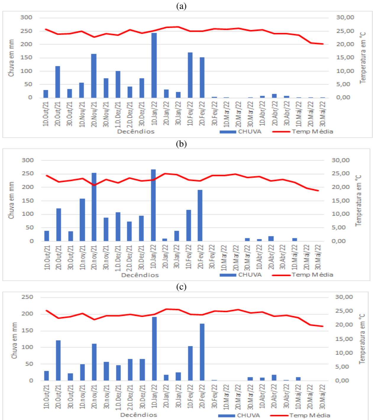
Figura 3: Histograma de Chuva e Temperatura: Caratinga (a); Timóteo (b) e PERD (c) – (outubro de 2021 a maio de 2022).
