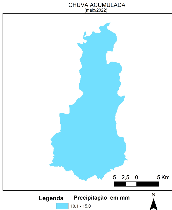
Figura 5 - Espacialização da Chuva da Acumulada em maio de 2022. FONTE dos Dados: INMET e INPE
