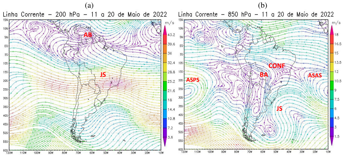
Figura 7 - Campos de Linha de Corrente 200 hPa - (a) e 850 hPa - (b), do 2º Decêndio de maio de 2022; demonstrando interação entre os sistemas atmosféricos: Alta da Bolívia (AB), Jato Subtropical (JS), Bloqueio Atmosférico (BA), Confluência (CONF), Anticiclone Subtropical do Atlântico Sul (ASAS) e o Anticiclone Subtropical do Pacífico Sul (ASPS).
